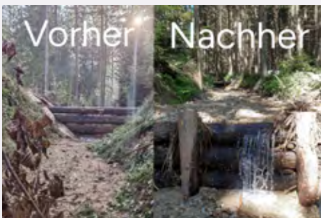
Kleinrückhaltebecken, Hochneukirchen
